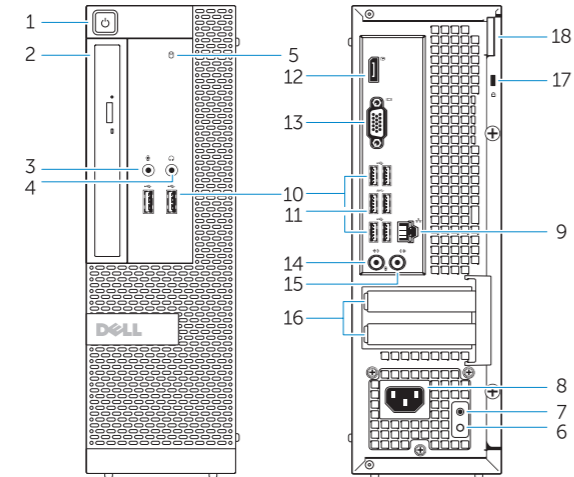
OptiPlex 3020 SFF
